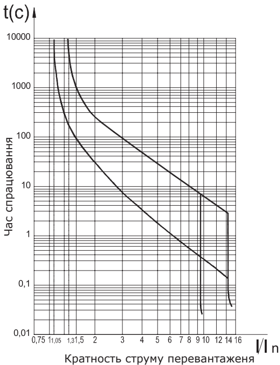
Рис. В.1 - Вимикачі з електромагнітними та тепловими розчеплювачами з уставкою по струму спрацювання 12 I_n при температурі 30^{\circ}C
