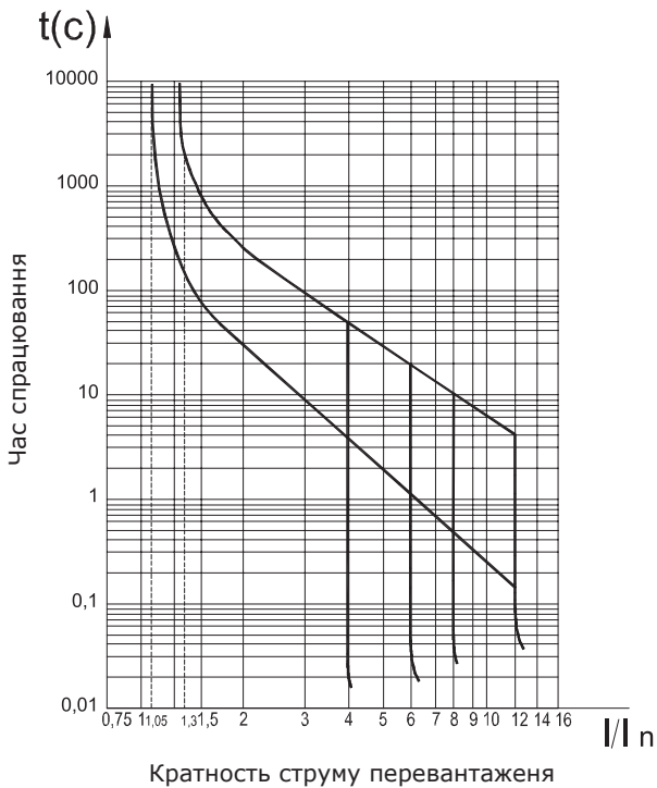
Рис. В.2 - Вимикачі з електромагнітними та тепловими розчеплювачами з уставкою по струму спрацювання 5I_n та 10I_n при температурі 30^\circ\text{C}
