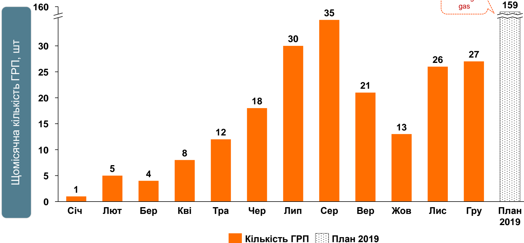
Кількість ГРП, шт
