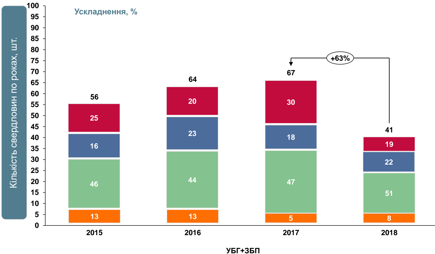
Розподіл ускладнень під час буріння від загальної кількості
